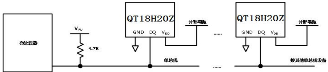
图 1：QT18H20Z 组网示意图
