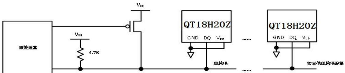
图 2：通过寄生电源供电
