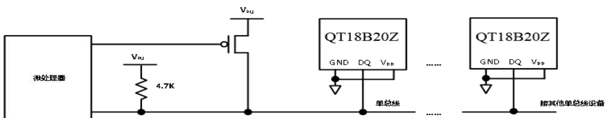
图 2：通过寄生电源供电
