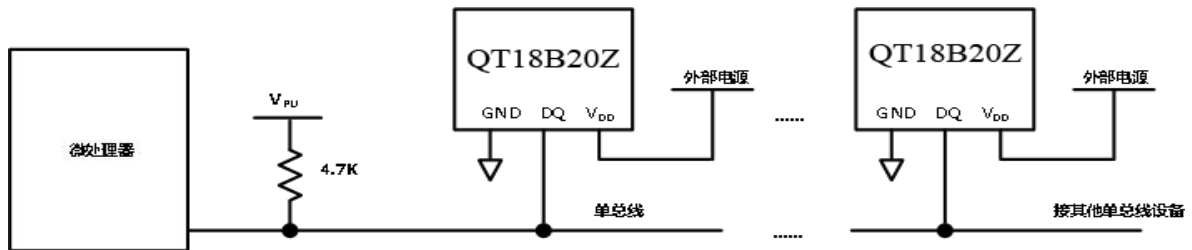
图 1：QT18B20Z 组网示意图
